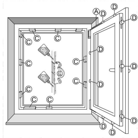
Schmierstellenübersicht
